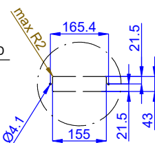
Dettaglio □ Scala 1:7
